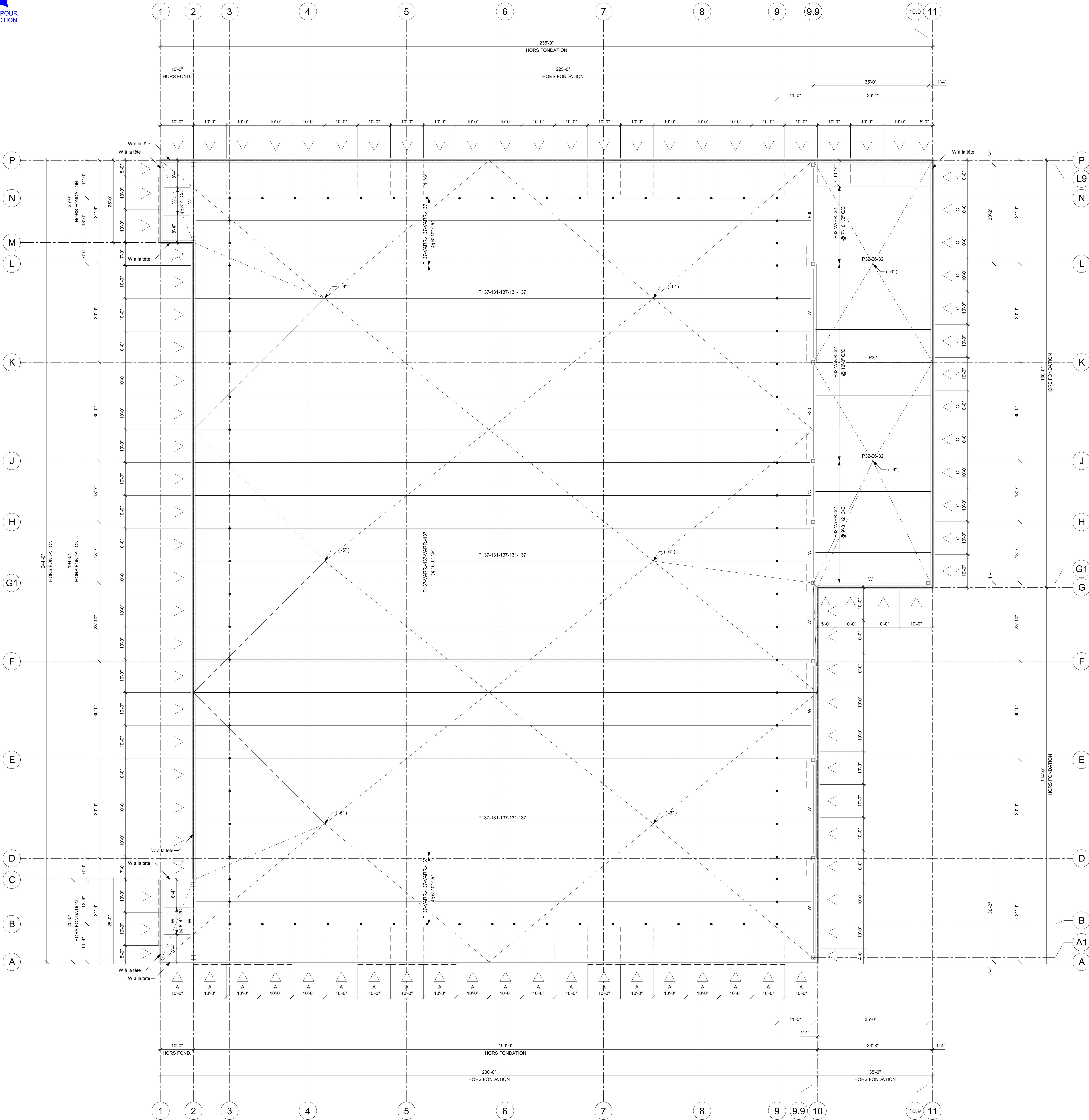
PLAN DE TOIT 3/32" = 1'-0"
