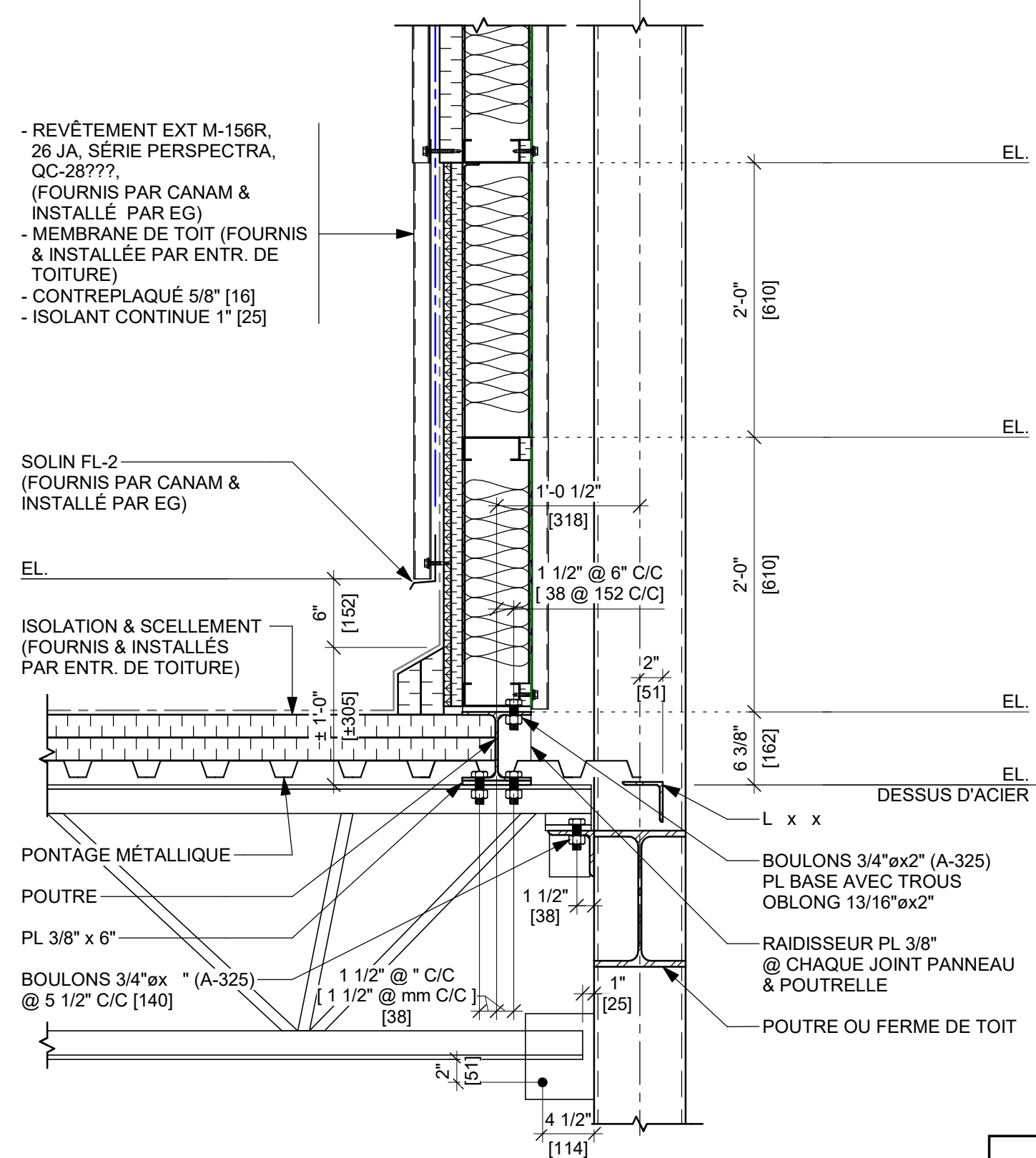
2 COUPE AXES 5 DE A @ B (OUEST) 3/32" = 1'-0"
